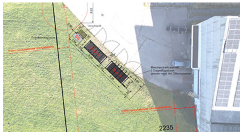
Lageplan Batteriespeicher auf der Parzelle 2235 im Eigentum der ews.
