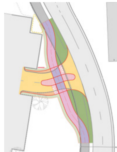
Plananschnitt «Veloroute Aldi Gloten».
